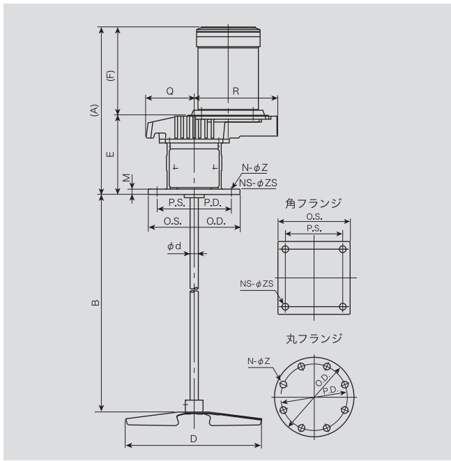
寸法図
