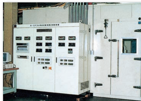
CO 2 対応カーエアコンベンチテスト装置 CO 2 Car Air Conditioner Bench Testing Device
